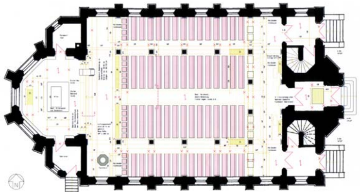
Grundriss EG
