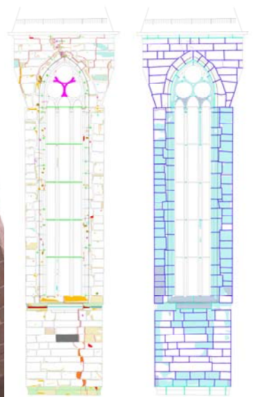
Schadenskartierung Chorfenster
