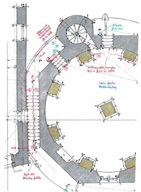
Schadenskartierung im „Glockenturm“ (Ausschnitt)
