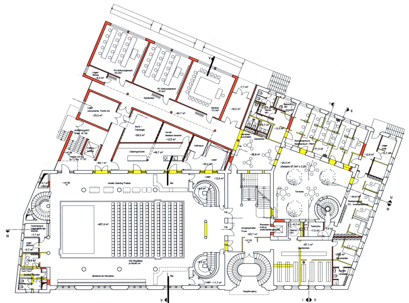
Grundriss Erdgeschoss
