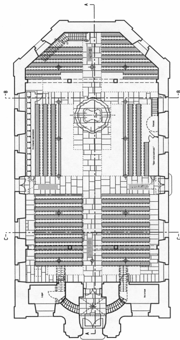
Grundriss
